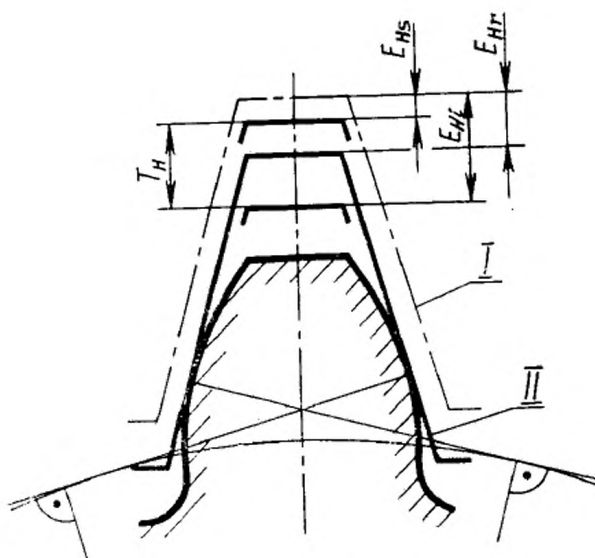
I—номинальное положение исходного контура; II—действительное положение исходного контура.
